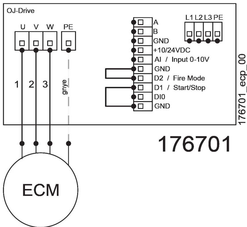
Anschluss 0-10V Signal
