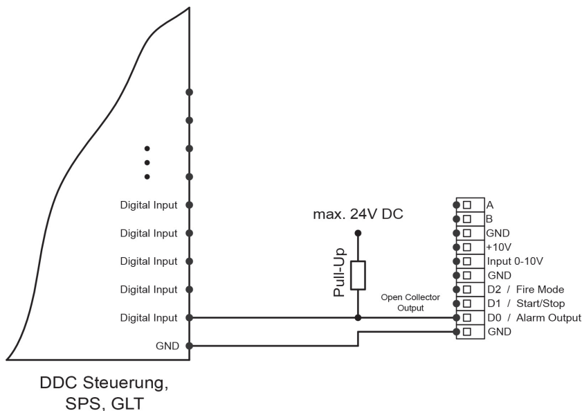
Alarmausgang auf Stererung aufgelegt
