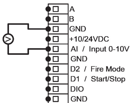
Anschluss 0-10V Signal
