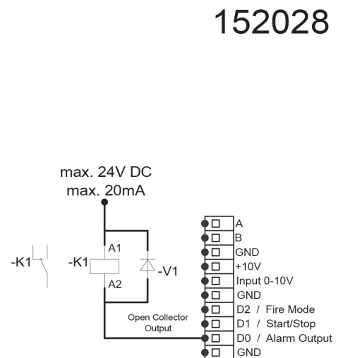
Relais mit Alarmausgang geschaltet
