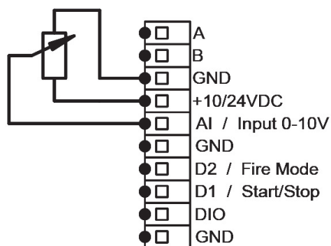
Anschluss Potentiometer
