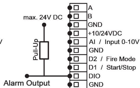
Anschluss Alarmausgang
